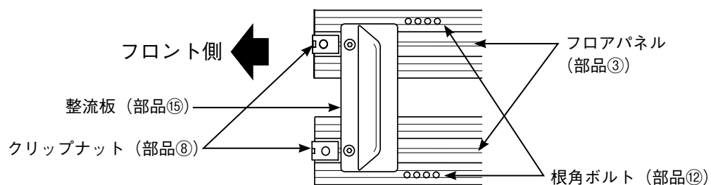
フロアパネルの組み立て完成図 (裏面から見た図)
